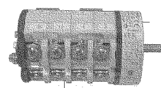
93.070 INTERRUPTEUR 32 A 0-1-2
