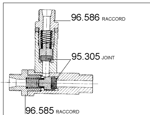
93.754 SOUPAPE DE SURPRESSION ET ANTI-RETOUR VERA
