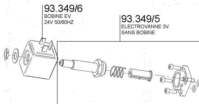
ELECTROVANNE VIDANGE ET CAPP.
