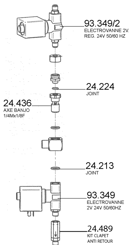
EV NETTOYAGES CAFE ET CAPP.
