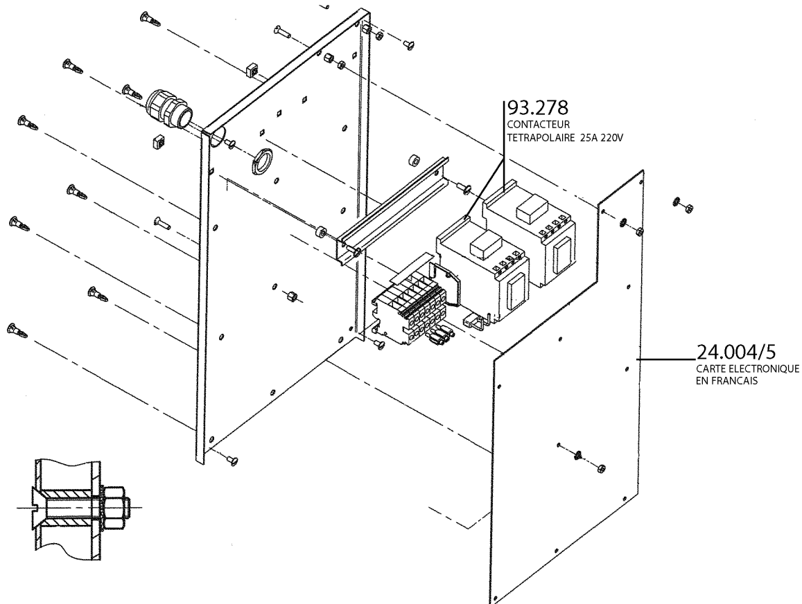
TABEAU DE RACCORDEMENT ELECTRIQUE
