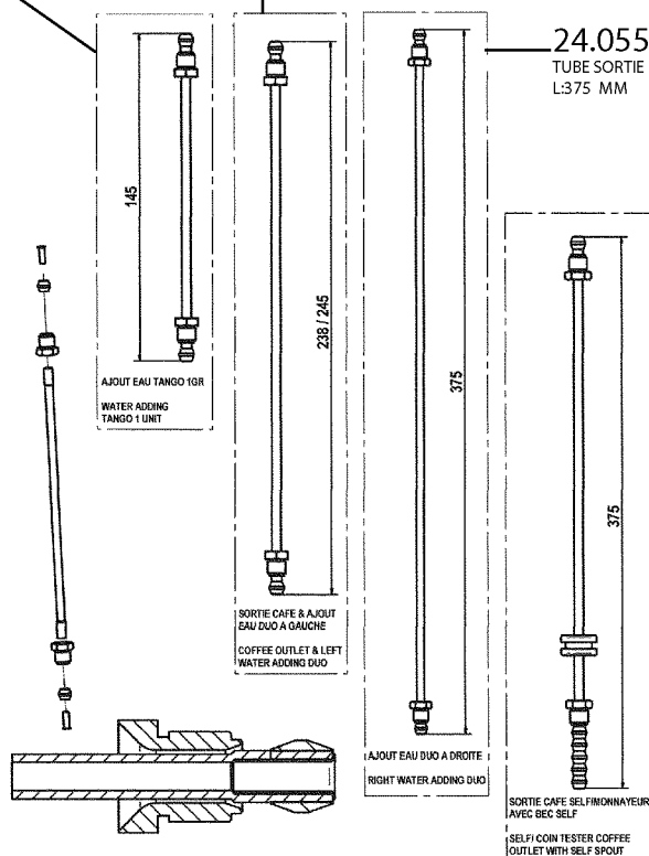
TUBE PTFE SORTIE CAFE ET EAU CHAUDE
