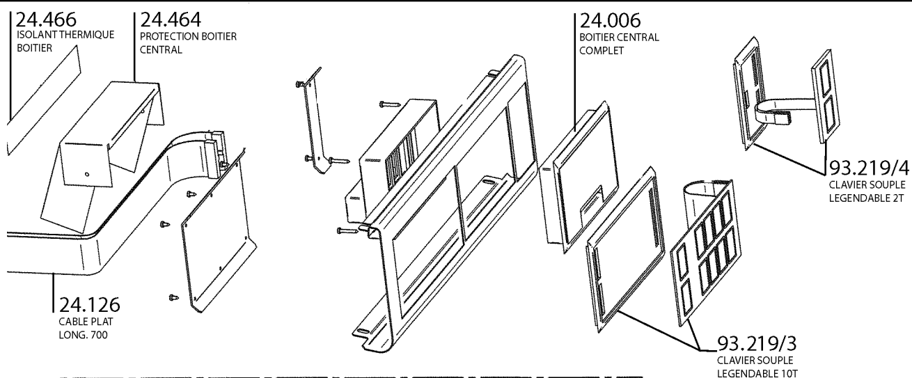
TABEAU DE RACCORDEMENT ELECTRIQUE
