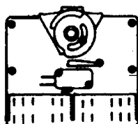
93.702 TYMER FIBER (FAEMA F/45)
