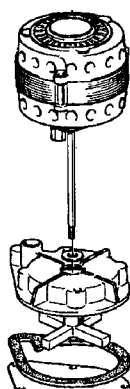
93.583 MOTEUR POMPE F15/30/45
